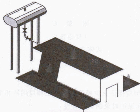
图 C.1 特高压换流变压器实体火灾模型示意图
