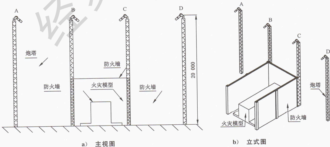
图 C.4 压缩空气泡沫消防炮布置图
