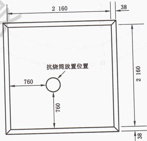
图 B.1 标准油盘火布置图
