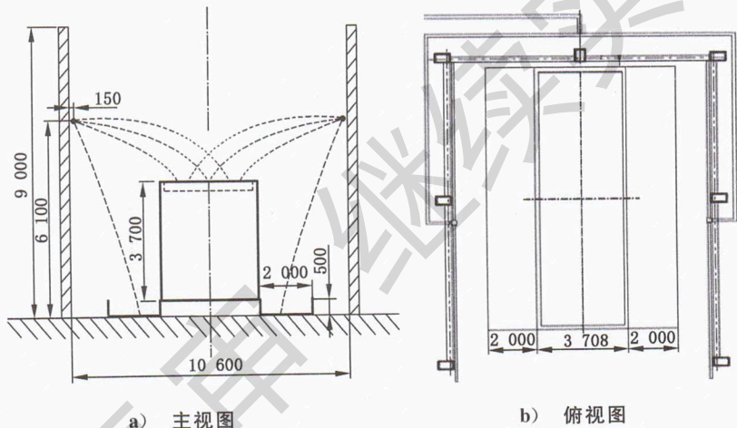
图 C.3 压缩空气泡沫喷淋管布置图
